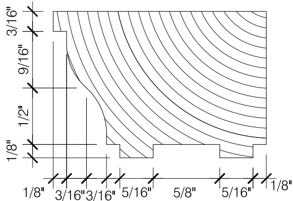
4 BRICK MOLD DETAIL SCALE: 3" = 1'-0"
