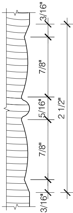
6 SCROLL WORK DETAIL SCALE: 3" = 1'-0"
