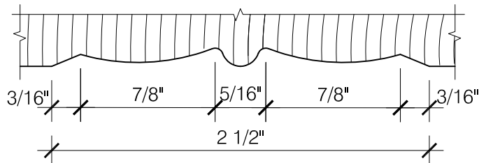
4 SCROLL WORK DETAIL SCALE: 3" = 1'-0"
