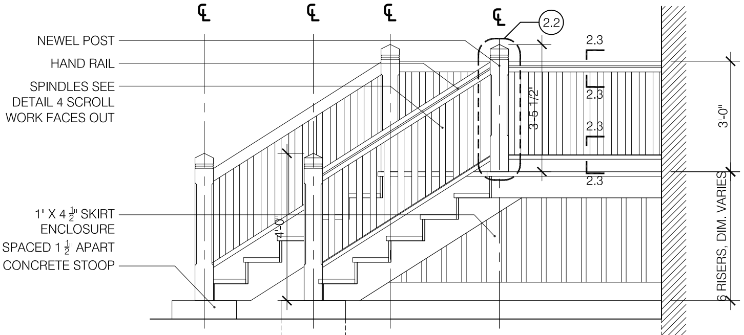
2.1 SIDE ELEVATION SCALE: 3/8" = 1'-0"
