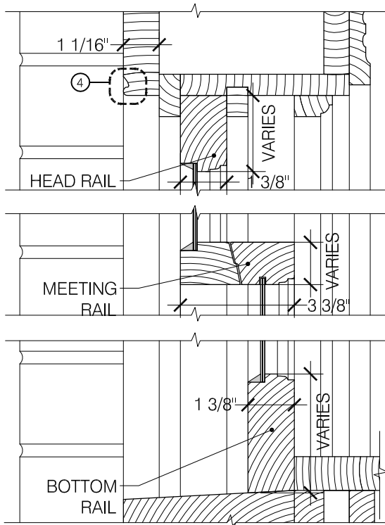
3 VERTICAL SECTION SCALE: 3" = 1'-0"
