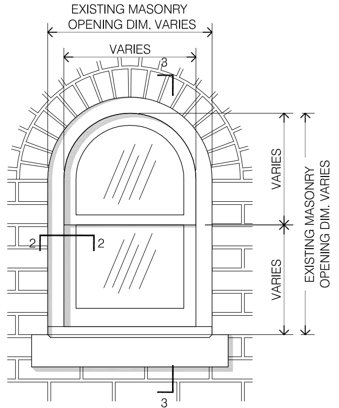
1 WINDOW ELEVATION SCALE: 1" = 1'-0"
