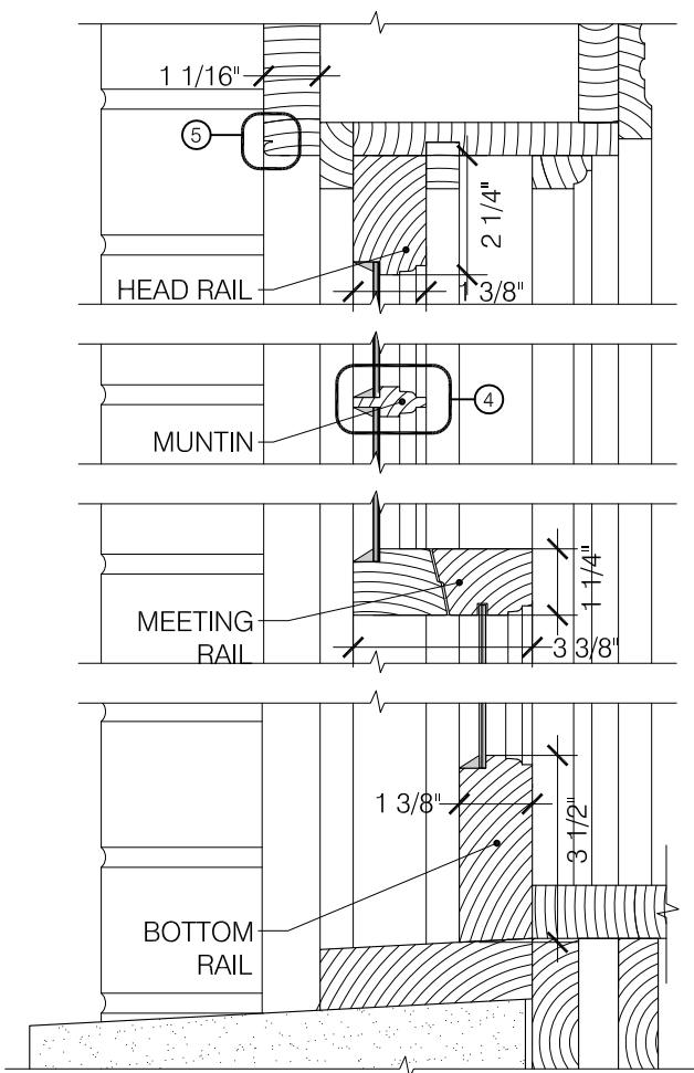
3 VERTICAL SECTION SCALE: 3" = 1'-0"
