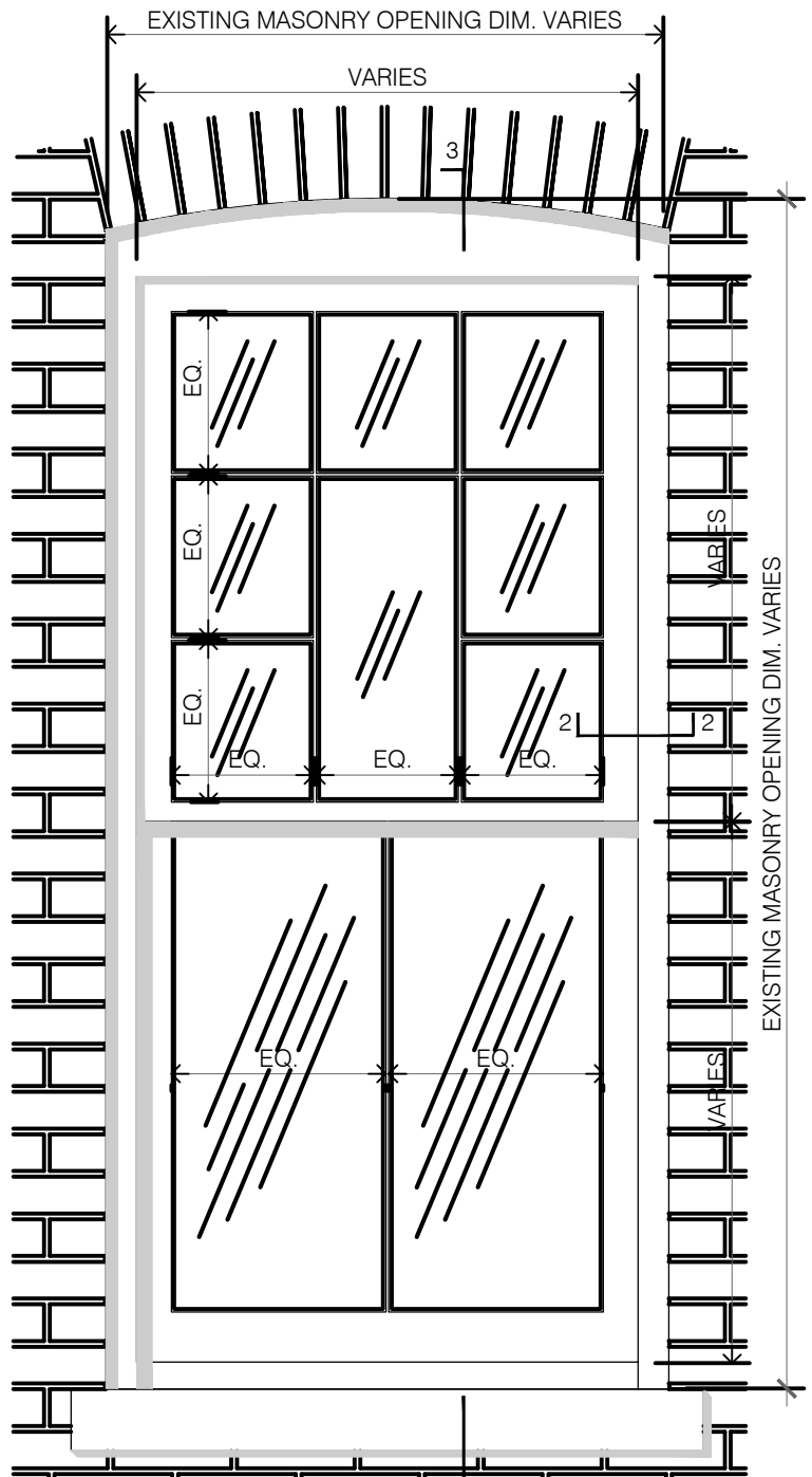
1 WINDOW ELEVATION SCALE: 1" = 1'-0"
