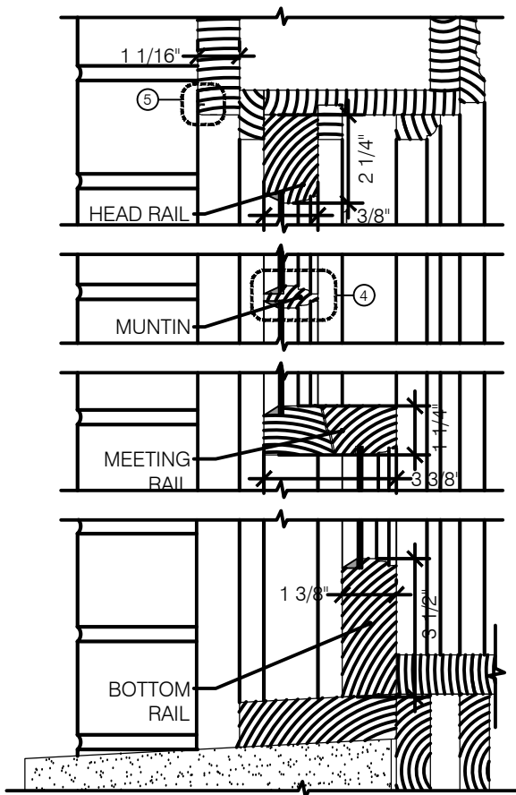
3 VERTICAL SECTION SCALE: 3" = 1'-0"
